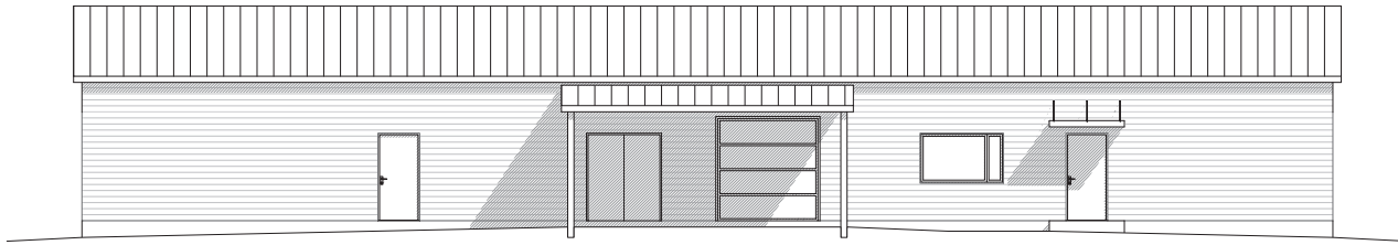
JULKISIVU LÄNTEEN/LOUNAASEEN
