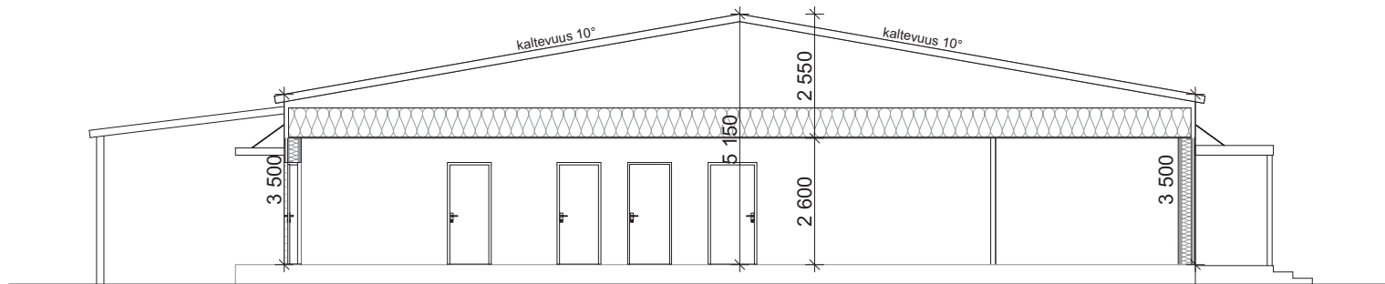
LEIKKAUS A-A
